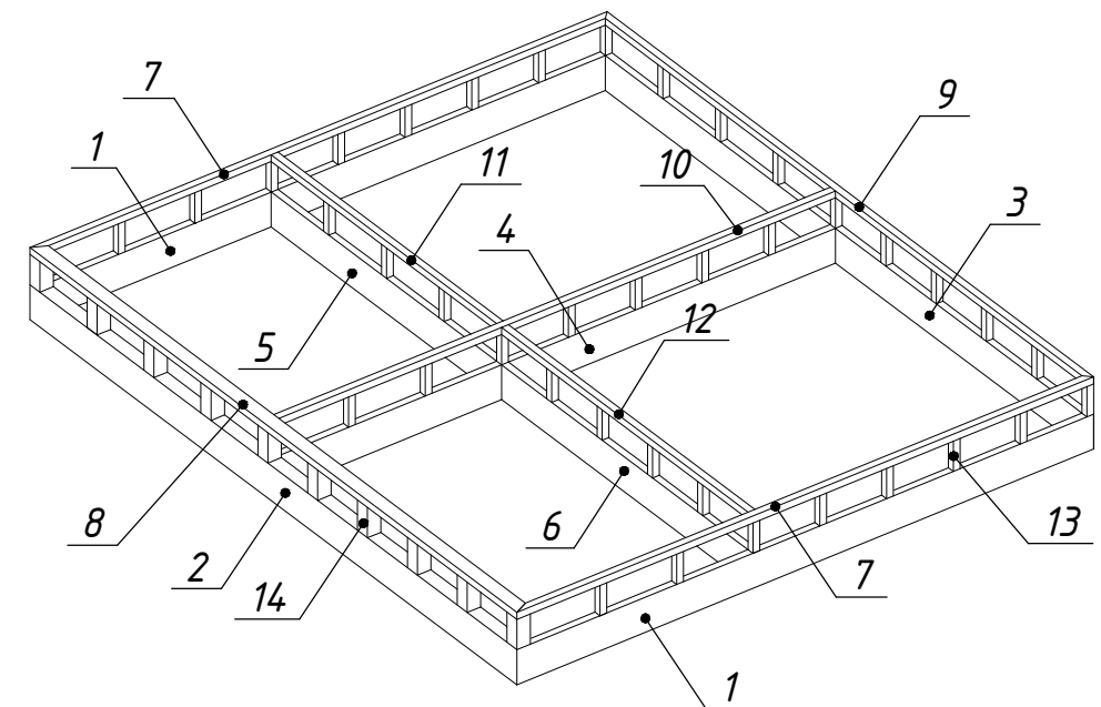
Изометрия представлена с тыльной стороны.
